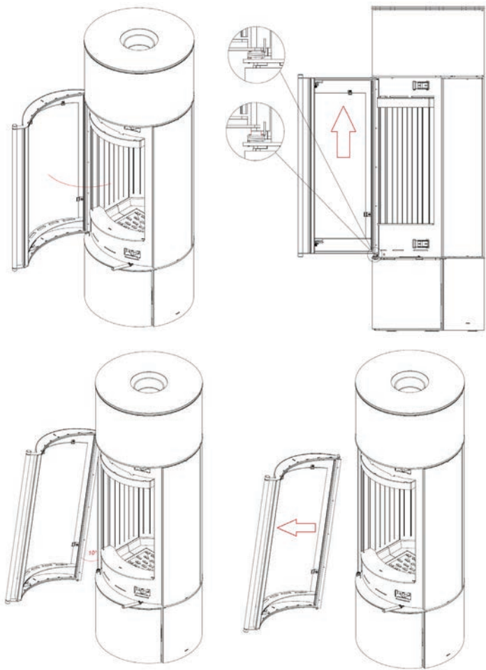
32. Schemat wymiany drzwi ANTARES. / 32. The ANTARES door-replacement diagram
