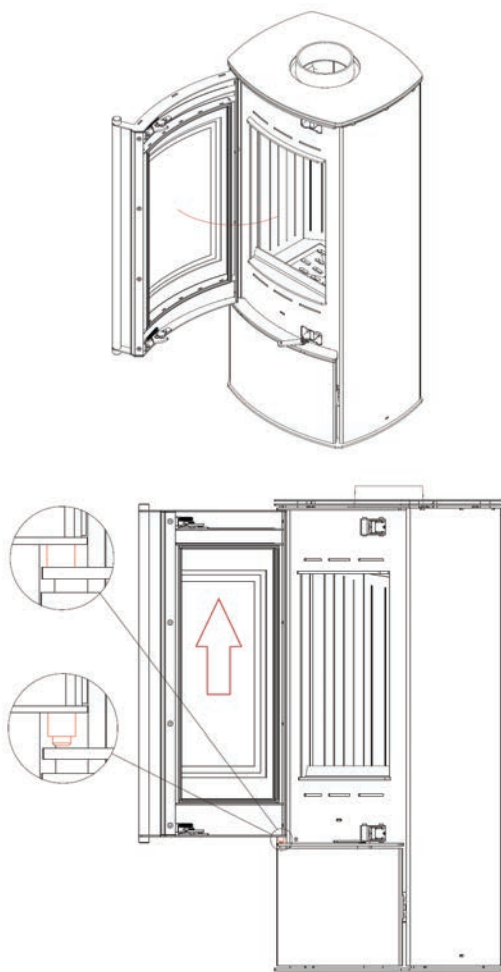
28. Schemat wymiany drzwi ATLAS. / The ATLAS door-replacement diagram
