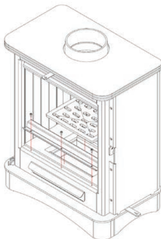
37. Kolejność demontażu oraz wymiany deflektora i wyłożenia accumotte – VEGA The procedure for the baffle and Accumotte lining disassembly and replacement – VEGA
